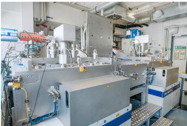
Abb. 2 CVD-Beschichtungsanlage (kurz für chemical vapour deposition) für die Funktionalisierung textiler Gewebe.
