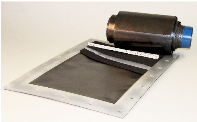
Abb. 2 2500 cm 2 Redox-Flow-Zelle und per Rolle-zu-Rolle-Verfahren gefertigte Bipolarplatte.
