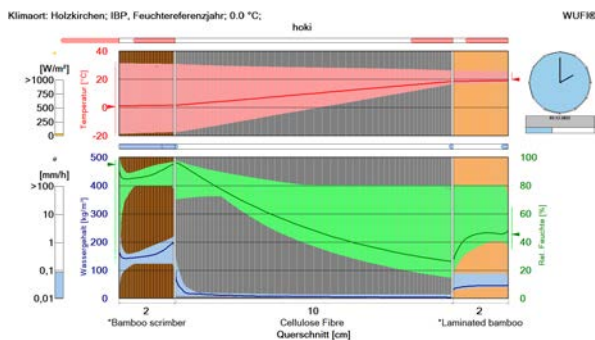
Abb. 2 Die Software WUFI® aus dem Fraunhofer IBP zeigt das Feuchteverhalten des Werkstoffs im zeitlichen Verlauf als Film an. Die Vertikalachse gibt Temperatur und Wassergehalt an, die Horizontalachse den Bauteilquerschnitt.
