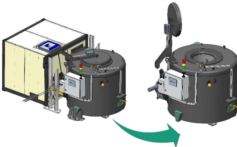
Bild 2: Mobile Tiegelpfanne mit Heat-Dock. Quelle: Fraunhofer IFF
