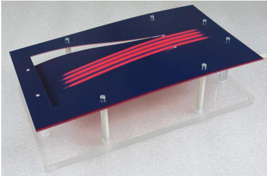
Bild 3, Demonstrator »Kühlluftklappe«: Formgedächtnis-Legierungen lassen sich einsetzen, um Lüftungssysteme für Motoren, Brennstoffzellen oder Batterien völlig autark arbeiten zu lassen. © Fraunhofer IWU | Bild in Farbe und Druckqualität: www.fraunhofer.de/presse .
